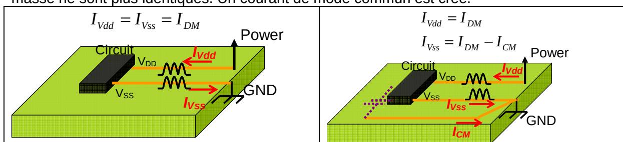
Figure 8 - Mode de circulation du courant – A gauche : mode différentiel, à droite : mode commun
