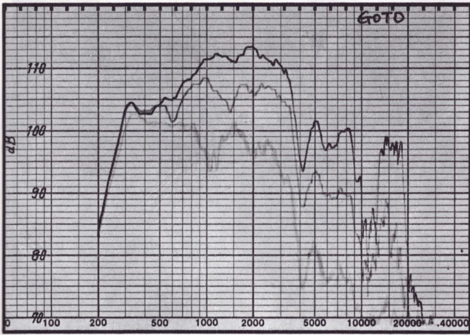
◇指向特性 (0°, 30°, 60°)
