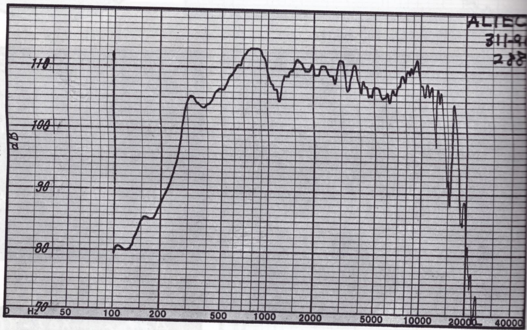
⇨ 周波数特性
